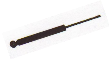
ALKO Auflaufdämpfer 2.8VB 351Z Gesamtlänge 605mm, Rohrlänge 440mm Durchmesser 29mm, Lochdurchmesser M14 Nr. 21726604 Miet-Lift Art.Nr. 53412
