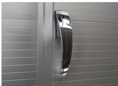
Türgriff zu Pferdeanhänger verschromt (Arizona WM Meyer) nicht verschliessbar ohne Zylinder, ohne Schlüssel. Totallänge 170mm Grundplatte 65x35mm. Ohne Innenverschluss
