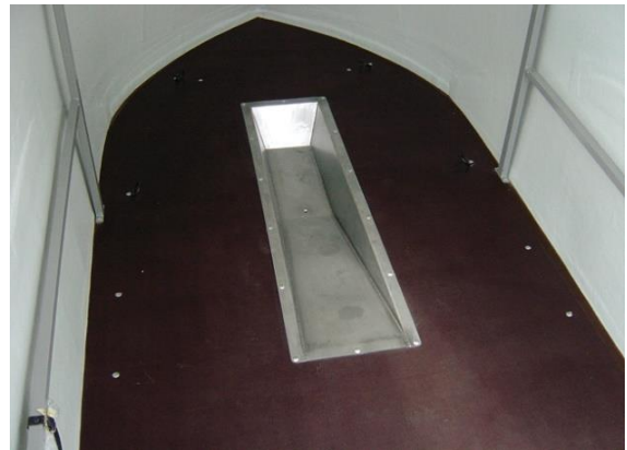
Motorradmulde 140 mittig montiert für Motorräder
