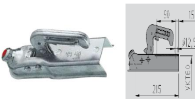
Kugelkupplung AK 7 Ausführung E Gesamtgewicht 750/800kg Anschluss 60mm vierkant Miet-Lift Art. Nr. 51005
