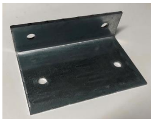
Befestigungsplatte für Klemmschelle Stahl verzinkt. Länge 150mm, Breite 100mm Winkel 50mm, Dicke 5mm. Lochabstand 105mm Lochabstand 105mm, Lochgrösse 11mm. Miet-Lift Art. Nr. 52128
