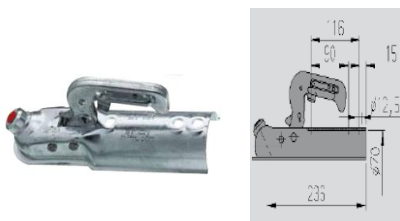
Kugelkupplung AK 7 Ausführung C Gesamtgewicht 750/800kg Anschluss 70mm rund Miet-Lift Art. Nr. 51002
