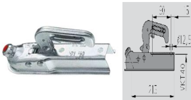
Kugelkupplung AK 7 Ausführung I Gesamtgewicht 750/800kg Anschluss 40mm vierkant Miet-Lift Art.Nr. 51006
