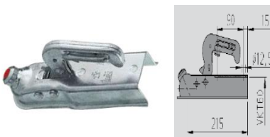
Kugelkupplung AK 7 Ausführung E Gesamtgewicht 750/800kg Anschluss 60mm vierkant Miet-Lift Art. Nr. 51005
