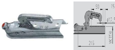
Kugelkupplung AK 7 Ausführung D Gesamtgewicht 750/800kg Anschluss 50mm vierkant Miet-Lift Art. Nr. 51004
