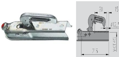
Kugelkupplung AK 7 Ausführung G Gesamtgewicht 750/800kg Anschluss 45mm vierkant Miet-Lift Art. Nr. 51003
