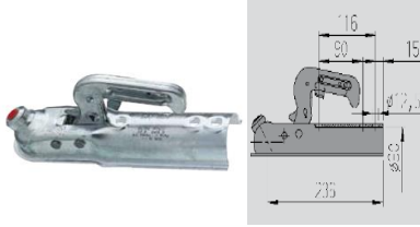
Kugelkupplung AK 7 Ausführung B Gesamtgewicht 750/800kg Anschluss 60mm rund Miet-Lift Art. Nr. 51001
